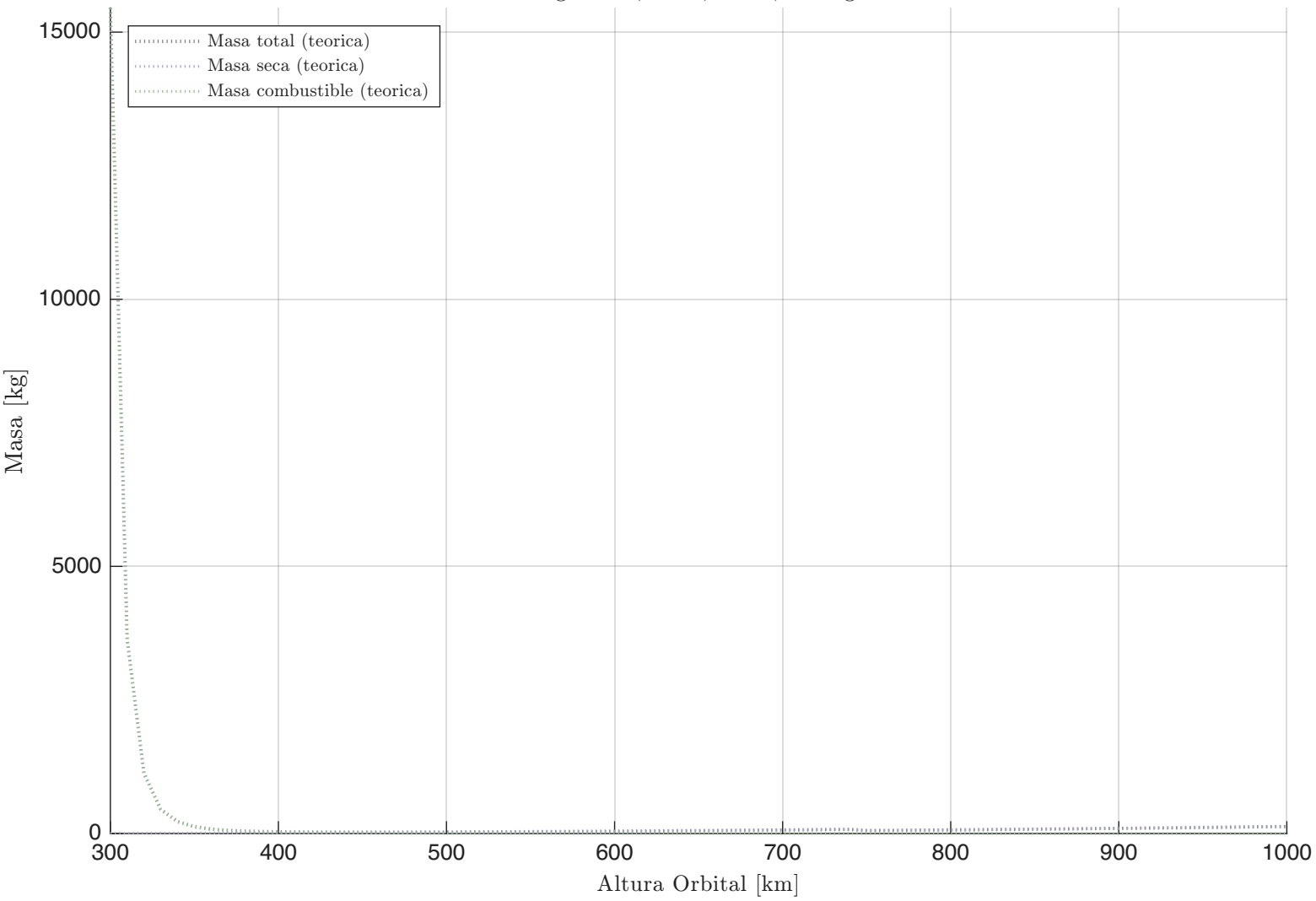
Desglose de Masas vs. Altura Config: 2 Sat, 1 Tel, Det 1, Cassegrain
